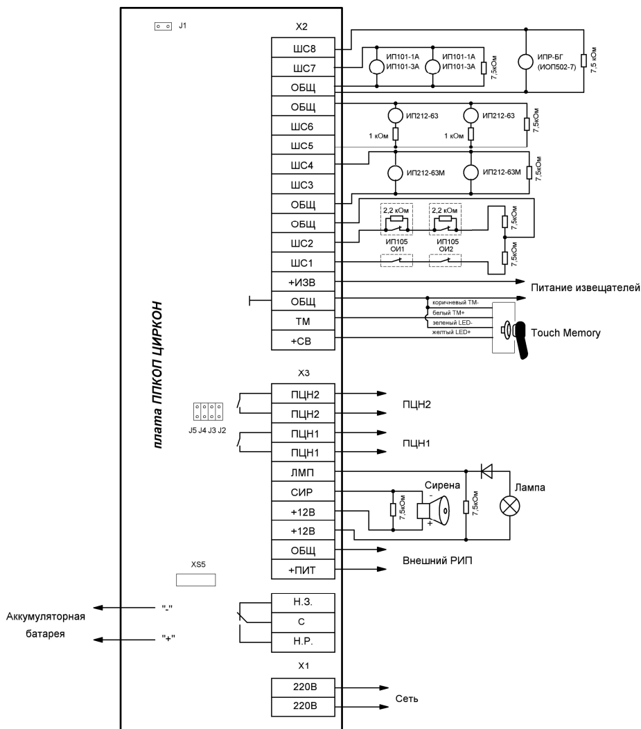
Рис. 1 Схема внешних соединений ППКОП «ЦИРКОН-8»
