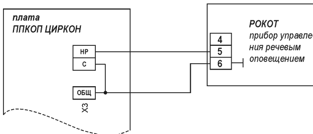
Рис. 5 Подключение прибора речевого оповещения «РОКОТ»
