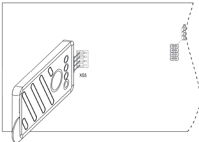
Рис. 8 Подключение USB-программатора к плате ППКОП «ЦИРКОН-3...-8»
