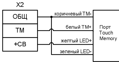
Рис. 2 Схема подключения порта Touch Memory к прибору
